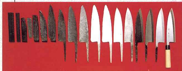
包丁の製造工程
