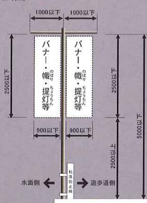
バナー寸法図
