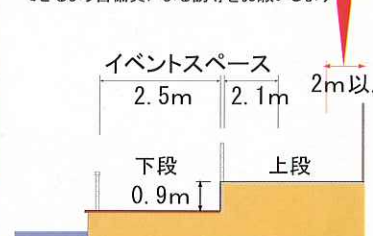
②-②断面図
